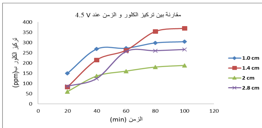
الشكل (3). العلاقة بين تركيز الكلور الحر بوحدة ppm وزمن التشغيل عند 4.5 V باستخدام أنود DSA
