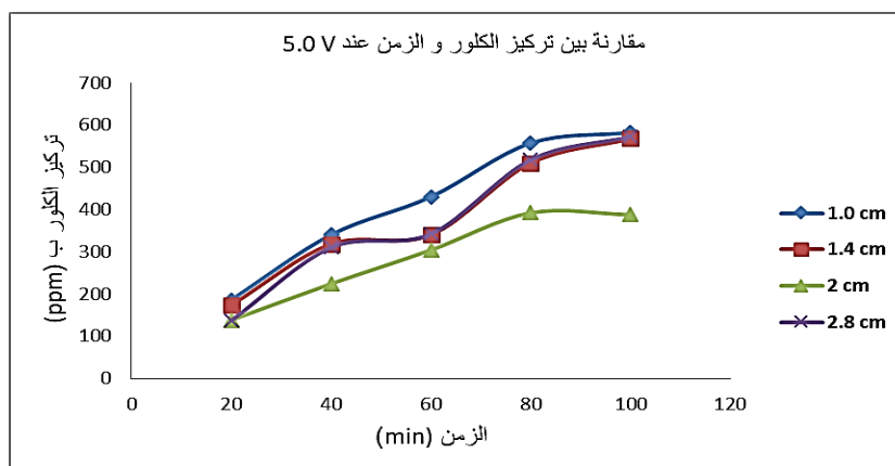
الشكل (4). العلاقة بين تركيز الكلور الحر بوحدة ppm وزمن التشغيل عند 5.0 V باستخدام أنود DSA
