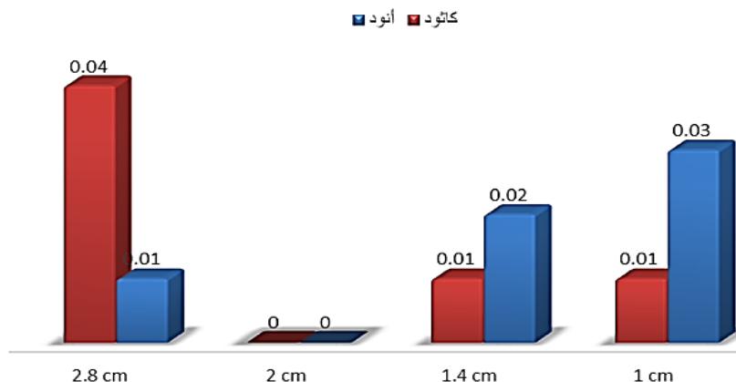
شكل (8). التغير الوزني للأنود والكاثود عند 5.0 V
